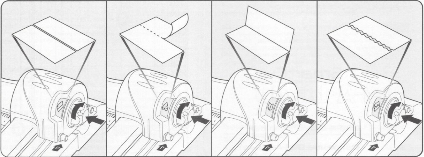
Selecting a Cutting Style Sélection d'un style de coupe Selección del estilo de corte
