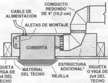
CUBIERTA MONTADA EN UNA VIGA DE 2x4 Se requiere una estructura adicional para las aletas de montaje. Descarga a 90° de las viguetas.
