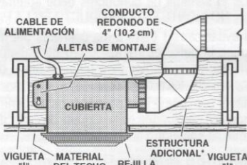
CUBIERTA MONTADA EN UNA VIGUETA "I" Se requiere una estructura adicional para las aletas de montaje. Descarga a 90° de las viguetas.
