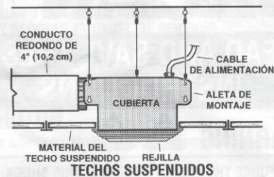
TECHOS SUSPENDIDOS Cubierta montada con cables. Montaje de tres puntos.
