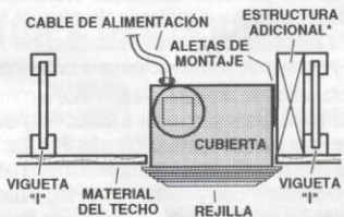
CUBIERTA MONTADA EN UNA VIGUETA "I" Se requiere una estructura adicional para las aletas de montaje. Descarga paralela a las viguetas.
