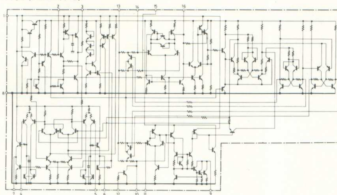
HA1196 (FM MPX IC)
